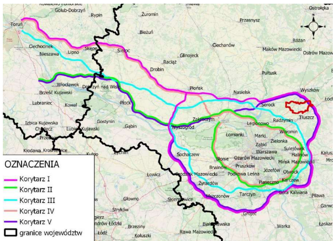
Schemat „Korytarze rozpatrywane w ramach Studium Sieciowego”, Streszczenie Studium korytarzowego dla inwestycji pod nazwą budowa drogi ekspresowej S10 Toruń (A1) – Warszawa (S8) wraz z budową Obwodnicy Aglomeracji Warszawskiej”, Warszawa, styczeń 2021 r.
