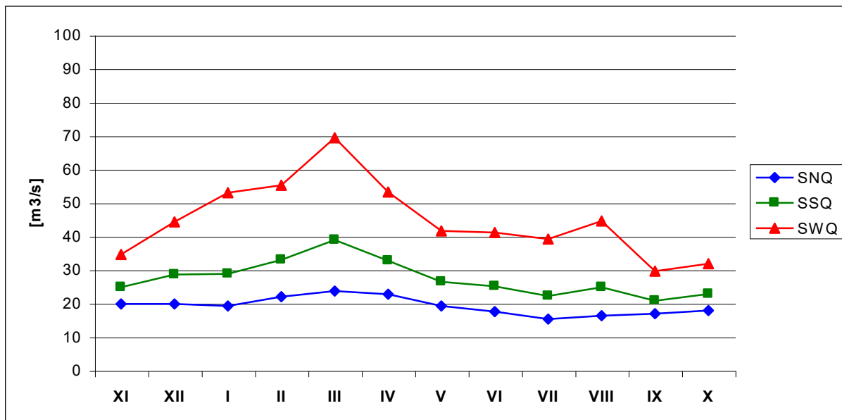
RYCINA 6: Gmina Wierzchlas – charakterystyczne przepływy miesięczne i roczne wody rzeki Warty ( \text{m}^3/\text{s} ) w okresie 1961 – 1991 na profilu Działoszyn.
