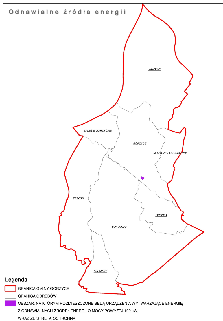
Ryc. 33. Lokalizacja OZE w Gorzycach. Źródło: opracowanie własne
