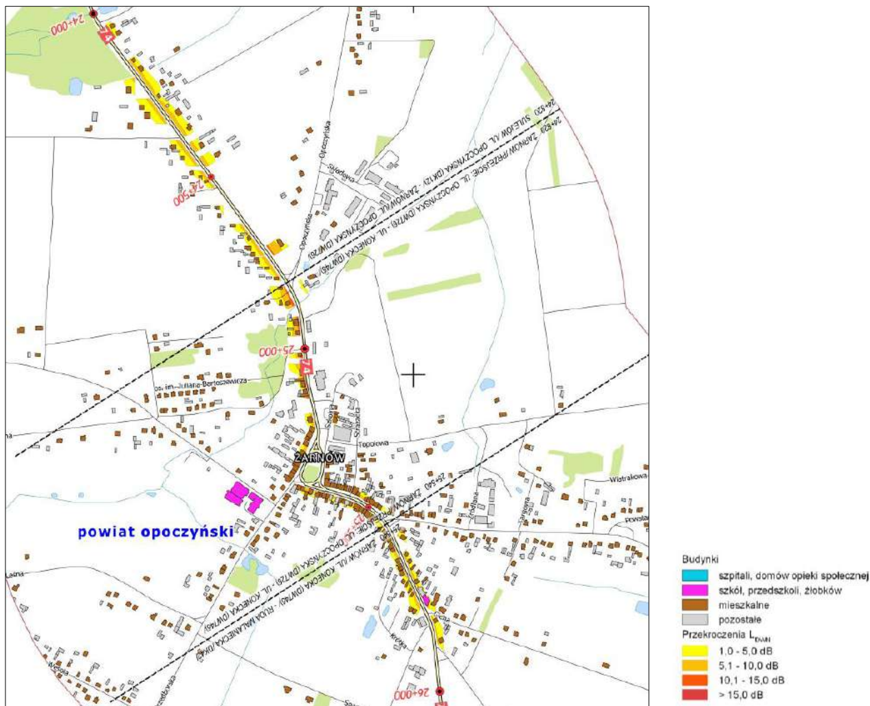
Ryc. 30. Przekroczenia dopuszczalnych źródeł hałasu wzdłuż drogi krajowej nr 64 w obszarze miejscowości Żarnów
