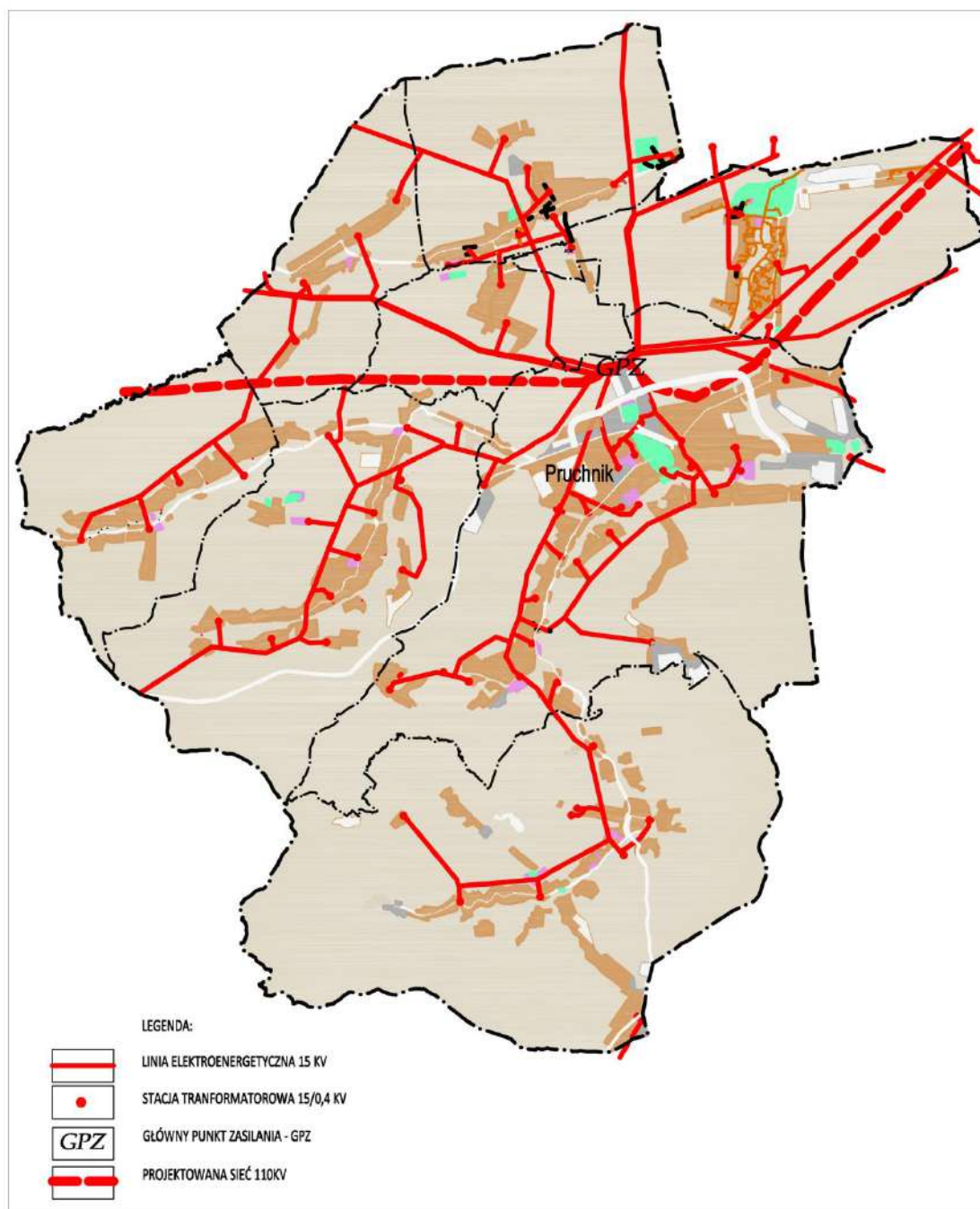
Schemat rozmieszczenia obiektów elektroenergetycznych
